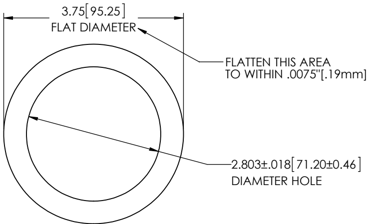
H.V. TANK HOLE DIMENSIONS
